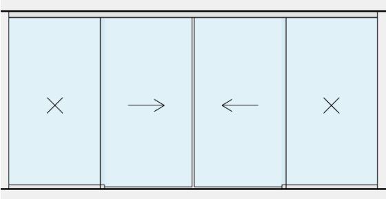
PUERTA DOBLE CON VIDRIO FIJO SINCRONIZADA
